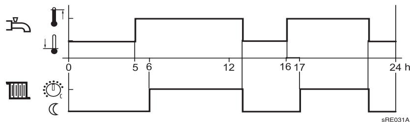
Fig. 11: liberar dependiendo de los programas temporizadores de los circuitos de calefacción (Ejemplo)
