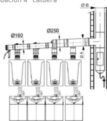
Diámetros de evacuación (A y B), según el nº de calderas en cascada y la longitud de la chimenea (H)
