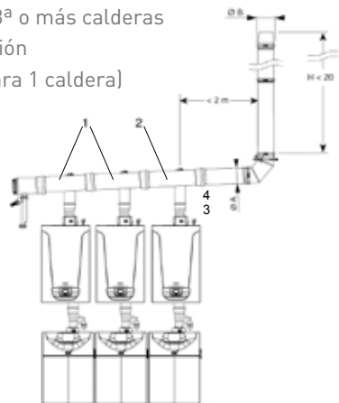
Diámetros de evacuación (A y B), según el nº de calderas en cascada y la longitud de la chimenea (H)
